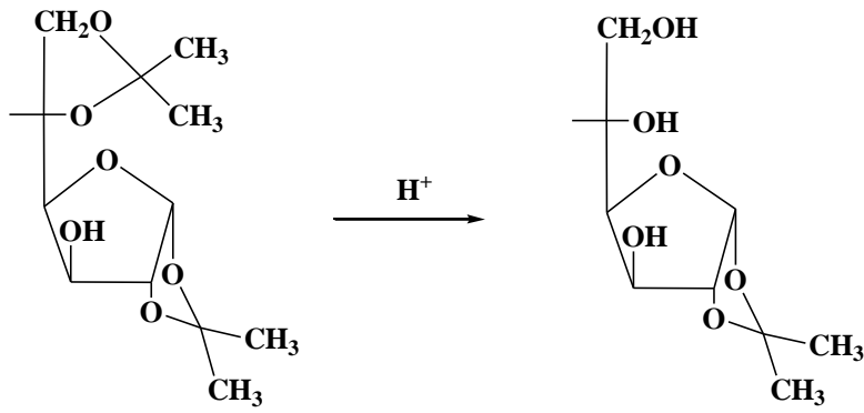
1,2-0-იზოპროპილიდენ- \alpha -D-გლუკოფურანოზა (მონოაცეტონგლუკოზა)
