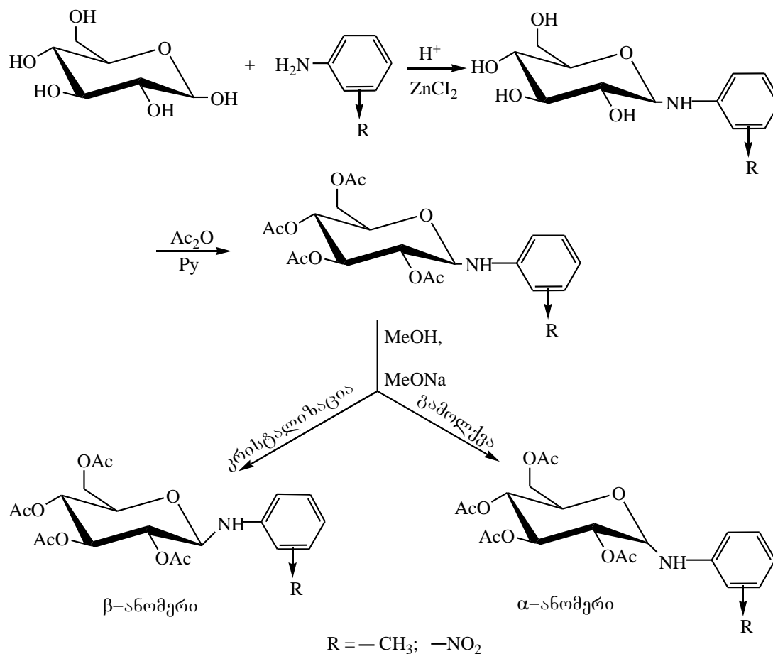
N-არილგლიკოზილამინების α და β ანომერების მიღების სქემა
